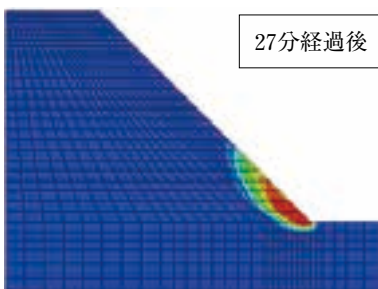
模型実験の解析結果の例、時間の進行に伴って赤で示された崩壊領域が拡大 One example of simulation result of the model test. The failure regions expressed by red expand with the elapsed times.
